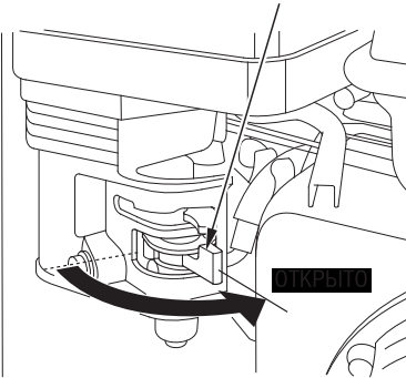
ЗАПОРНЫЙ КРАН ТЮПЛИПРОВОДА
