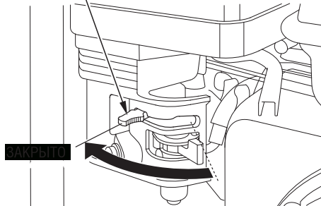
РЫЧАГ УПРАВЛЕНИЯ ВОЗДУШНОЙ ЗАСЛОНКОЙ
